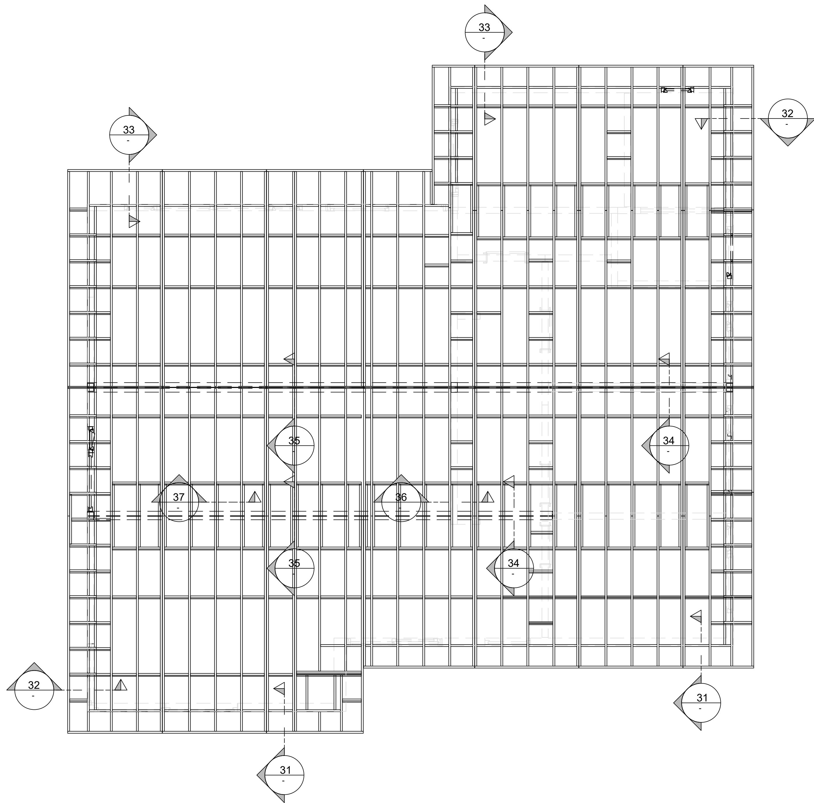
GRUNNMYND, ÞAK - EININGAR 1:50
