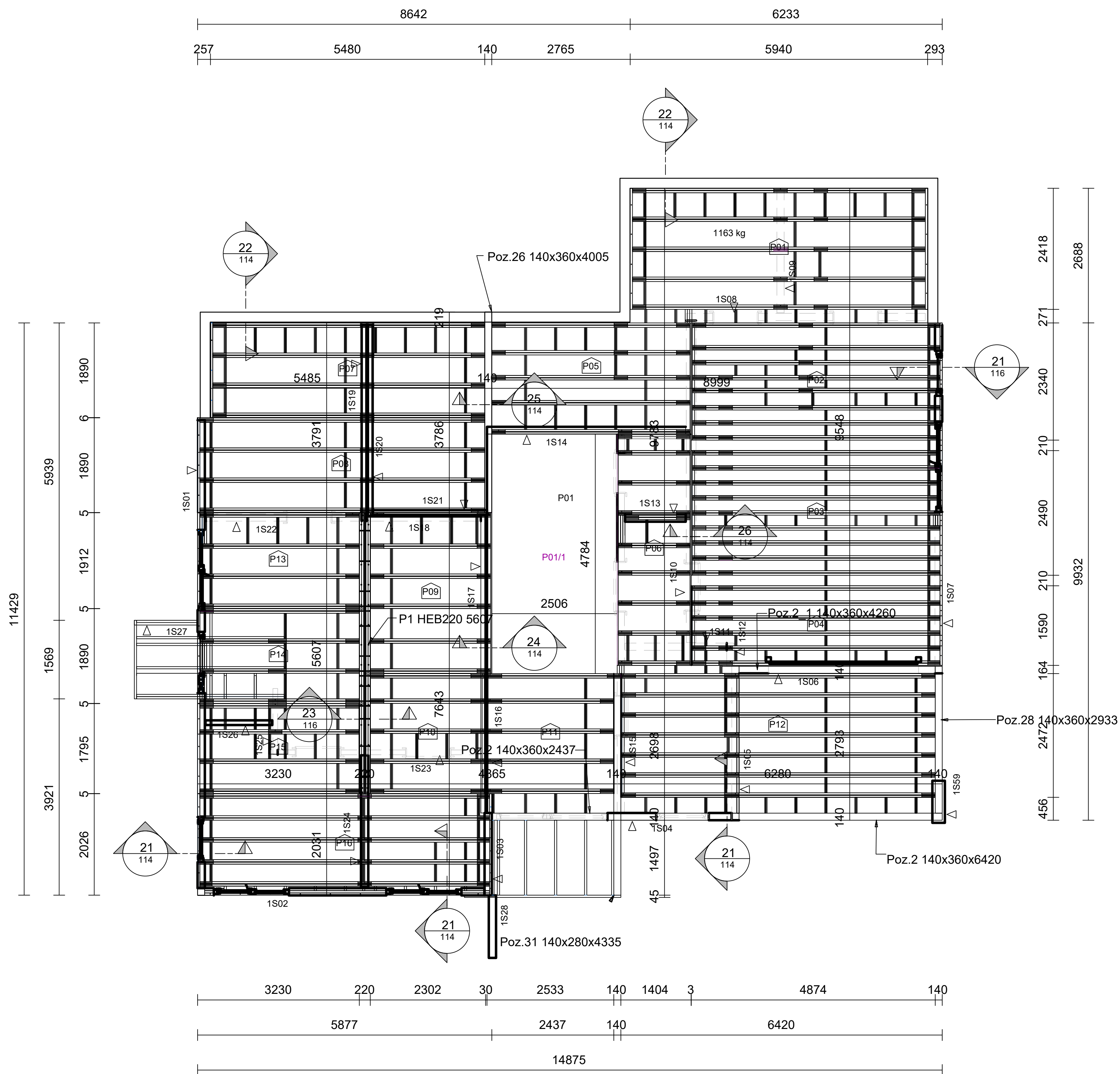
GRUNNMYND, 2.HÆÐ - ÚTVEGGIR - GÓLFEININGAR 1:50
