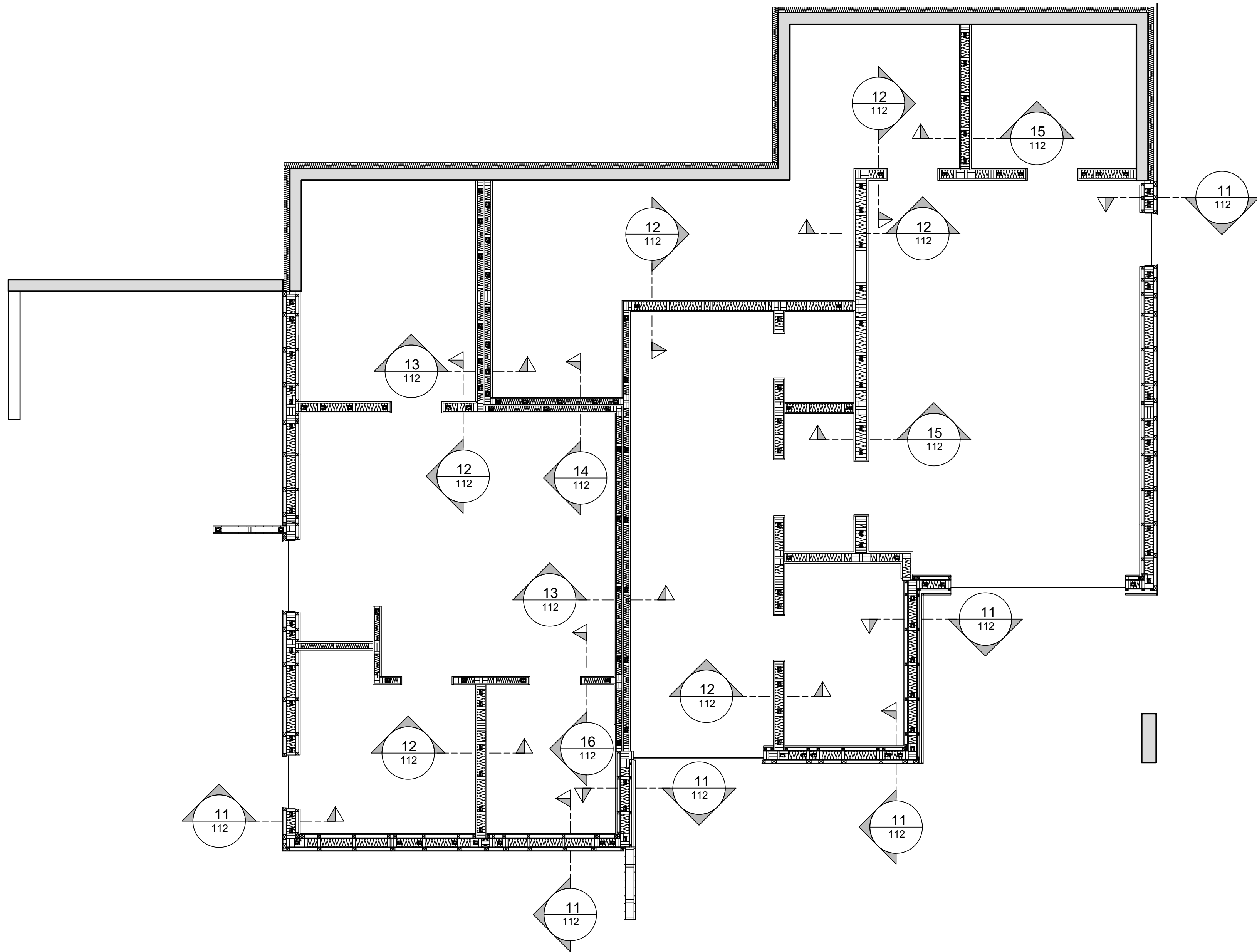
GRUNNMYND, 1.HÆÐ - FESTINGAR VEGGEININGA 1:50
